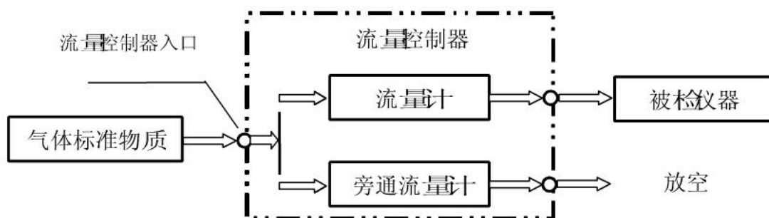
图 1 流量控制器
